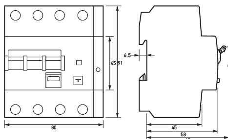
Maßzeichnung FI-/LS-Kombinationen DRCBO 4 Co6/o,10/3N-B+
