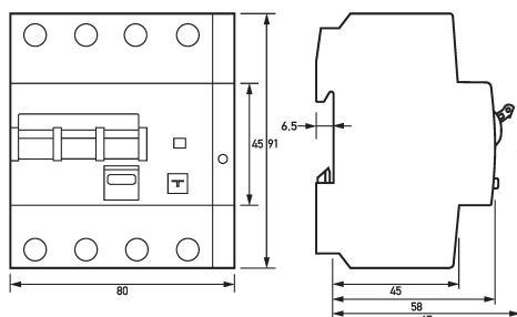
Maßzeichnung FI-/LS-Kombinationen DRCBO 4 C13/0,30/3N-B+
