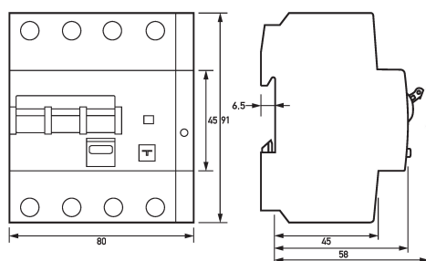
Maßzeichnung FI-/LS-Kombinationen DRCBO 4 C10/0,30/3N-B+
