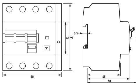
Maßzeichnung FI-/LS-Kombinationen DRCBO 4 Co6/0,30/3N-B+
