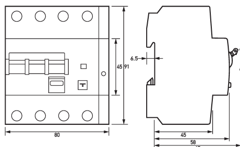
Maßzeichnung FI-/LS-Kombinationen DRCBO 4 B25/0,30/3N-B+
