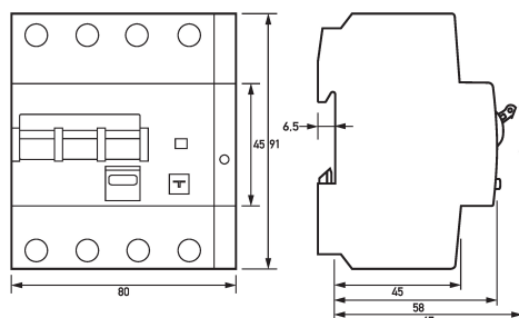
Maßzeichnung FI-/LS-Kombinationen DRCBO 4 B16/0,03/3N-B+
