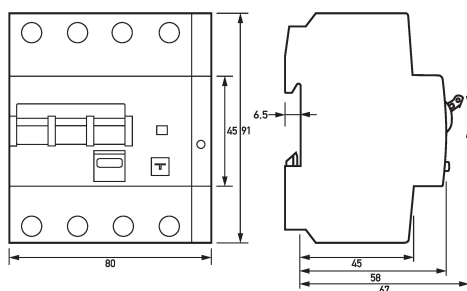
Maßzeichnung FI-/LS-Kombinationen DRCBO 4 C13/0,10/3N-B NK
