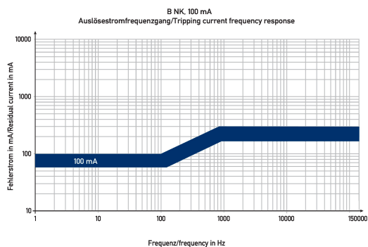
Diagramme FI-/LS-Kombinationen DRCBO 4 C10/0,10/3N-B NK
