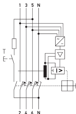
Schaltungsbeispiel FI-/LS-Kombinationen DRCBO 4 B20/0,10/3N-B NK
