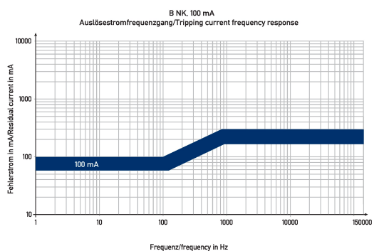
Diagramme FI-/LS-Kombinationen DRCBO 4 B16/0,10/3N-B NK
