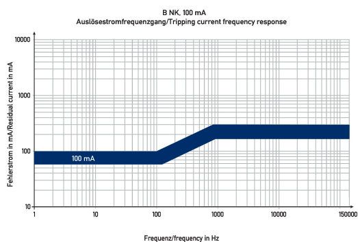
Diagramme FI-/LS-Kombinationen DRCBO 4 B10/0,10/3N-B NK
