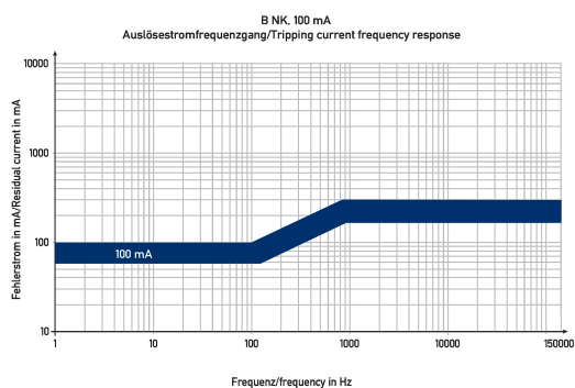
Diagramme FI-/LS-Kombinationen DRCBO 4 Bo6/0,10/3N-B NK
