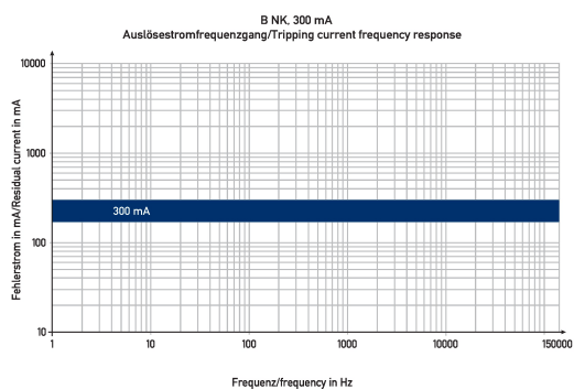
Diagramme FI-/LS-Kombinationen DRCBO 4 C32/0,30/3N-B NK
