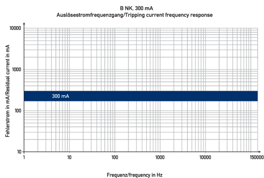
Diagramme FI-/LS-Kombinationen DRCBO 4 C13/0,30/3N-B NK
