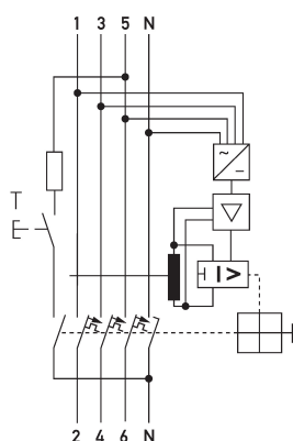
Schaltungsbeispiel FI-/LS-Kombinationen DRCBO 4 C13/0,30/3N-B NK
