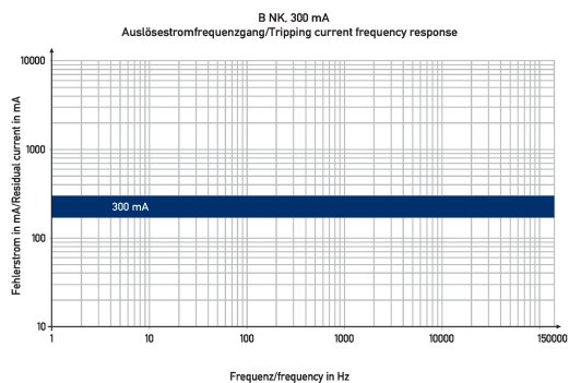
Diagramme FI-/LS-Kombinationen DRCBO 4 C10/0,30/3N-B NK
