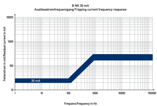
Diagramme FI-/LS-Kombinationen DRCBO 4 C32/0,03/3N-B NK
