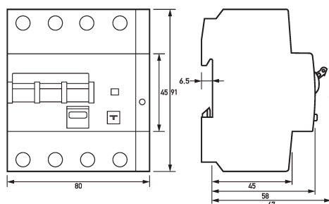
Maßzeichnung FI-/LS-Kombinationen DRCBO 4 C10/0,03/3N-B NK
