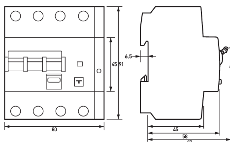
Maßzeichnung FI-/LS-Kombinationen DRCBO 4 Co6/o,03/3N-B NK
