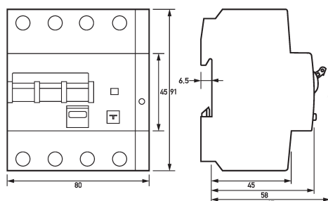
Maßzeichnung FI-/LS-Kombinationen DRCBO 4 B25/0,30/3N-B NK
