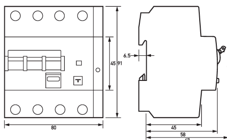
Maßzeichnung FI-/LS-Kombinationen DRCBO 4 B20/0,30/3N-B NK
