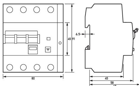
Maßzeichnung FI-/LS-Kombinationen DRCBO 4 B13/0,30/3N-B NK
