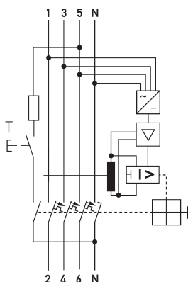
Schaltungsbeispiel FI-/LS-Kombinationen DRCBO 4 Bo6/o,3o/3N-B NK
