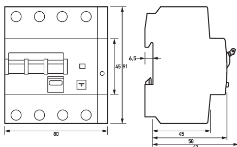
Maßzeichnung FI-/LS-Kombinationen DRCBO 4 Bo6/o,3o/3N-B NK
