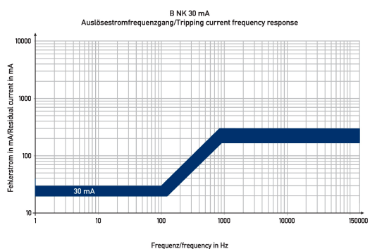
Diagramme FI-/LS-Kombinationen DRCBO 4 B20/0,03/3N-B NK
