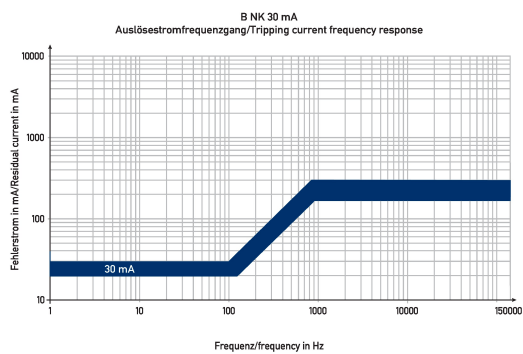
Diagramme FI-/LS-Kombinationen DRCBO 4 B13/0,03/3N-B NK
