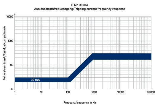
Diagramme FI-/LS-Kombinationen DRCBO 4 B10/0,03/3N-B NK
