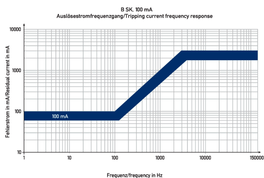
Diagramme FI-/LS-Kombinationen DRCBO 4 C32/0,10/3N-B SK
