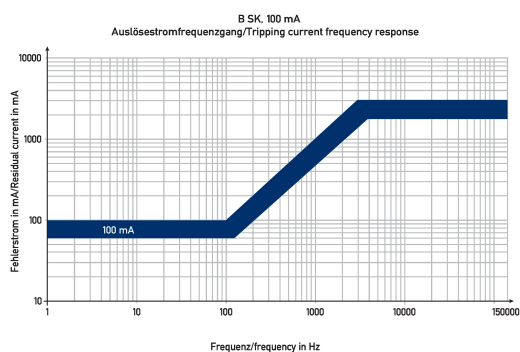
Diagramme FI-/LS-Kombinationen DRCBO 4 C16/0,10/3N-B SK
