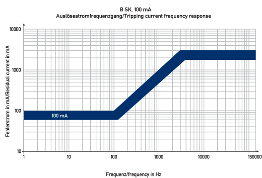
Diagramme FI-/LS-Kombinationen DRCBO 4 B20/0,10/3N-B SK
