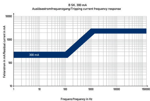
Diagramme FI-/LS-Kombinationen DRCBO 4 C32/0,30/3N-B SK
