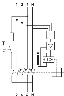
Schaltungsbeispiel FI-/LS-Kombinationen DRCBO 4 C32/0,30/3N-B SK
