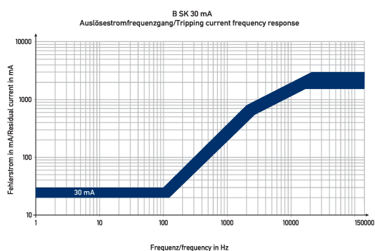
Diagramme FI-/LS-Kombinationen DRCBO 4 C16/0,03/3N-B SK
