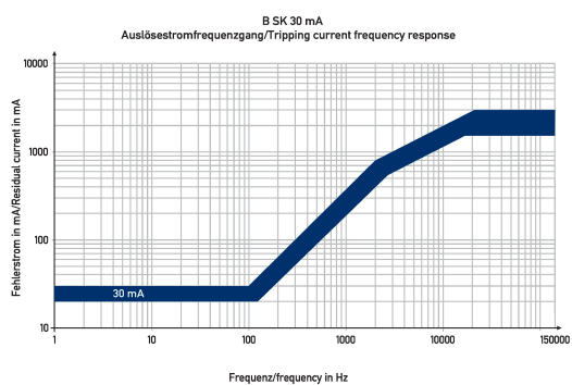
Diagramme FI-/LS-Kombinationen DRCBO 4 C13/0,03/3N-B SK
