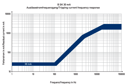
Diagramme FI-/LS-Kombinationen DRCBO 4 B16/0,03/3N-B SK
