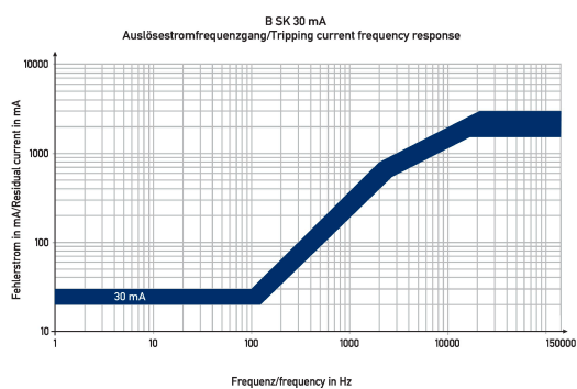
Diagramme FI-/LS-Kombinationen DRCBO 4 B13/0,03/3N-B SK
