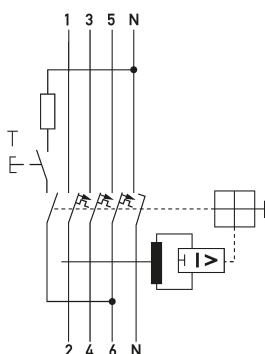
Schaltungsbeispiel FI-/LS-Kombinationen DRCBO 4 C13/0,30/3N-A
