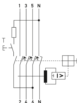
Schaltungsbeispiel FI-/LS-Kombinationen DRCBO 4 C10/0,30/3N-A
