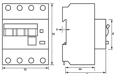
Maßzeichnung FI-/LS-Kombinationen DRCBO 4 Co6/0,30/3N-A
