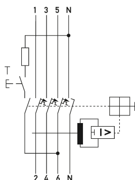
Schaltungsbeispiel FI-/LS-Kombinationen DRCBO 4 C13/0,03/3N-A
