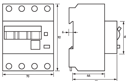
Maßzeichnung FI-/LS-Kombinationen DRCBO 4 C13/0,03/3N-A
