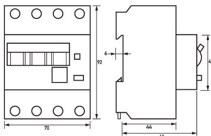
Maßzeichnung FI-/LS-Kombinationen DRCBO 4 B32/0,30/3N-A
