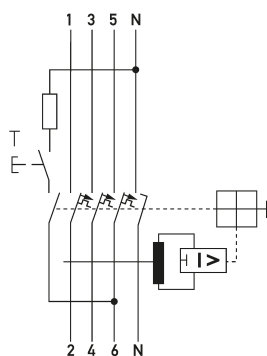
Schaltungsbeispiel FI-/LS-Kombinationen DRCBO 4 B20/0,30/3N-A
