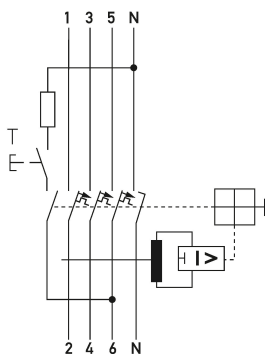
Schaltungsbeispiel FI-/LS-Kombinationen DRCBO 4 B13/0,30/3N-A
