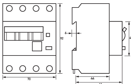
Maßzeichnung FI-/LS-Kombinationen DRCBO 4 Bo6/0,30/3N-A
