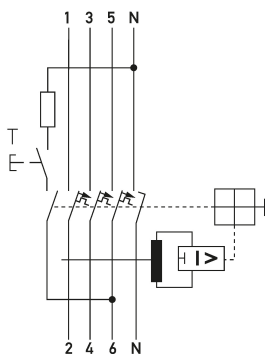
Schaltungsbeispiel FI-/LS-Kombinationen DRCBO 4 B20/0,03/3N-A
