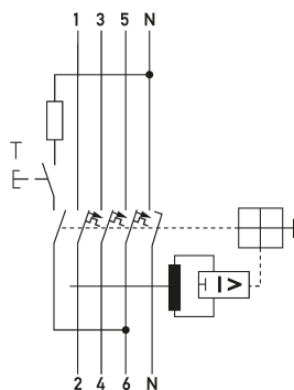
Schaltungsbeispiel FI-/LS-Kombinationen DRCBO 4 B13/0,03/3N-A
