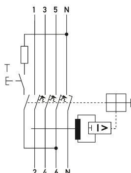
Schaltungsbeispiel FI-/LS-Kombinationen DRCBO 4 Bo6/0,03/3N-A
