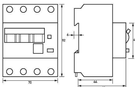
Maßzeichnung FI-/LS-Kombinationen DRCBO 4 Bo6/0,03/3N-A
