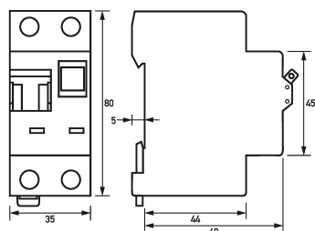
Maßzeichnung FI-/LS-Kombinationen DRCBO 3 C25/0,30/1N-A
