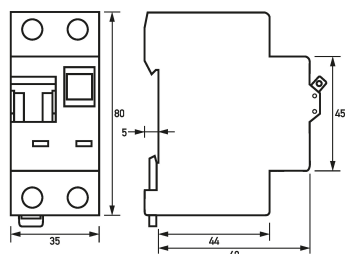
Maßzeichnung FI-/LS-Kombinationen DRCBO 3 C20/0,30/1N-A
