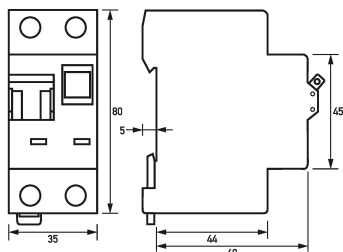
Maßzeichnung FI-/LS-Kombinationen DRCBO 3 B32/0,30/1N-A
