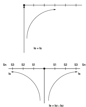
Diagramme Verdrahtungsmaterial BG4.3.10
