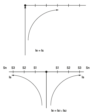
Diagramme Verdrahtungsmaterial BG4.5.16
