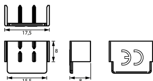
Maßzeichnung Endkappen EK-3/10/16
